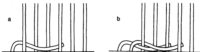
Zavírka jednoduchá s konci dovnitř a, b) za jeden osnovní prut, přes dva a dovnitř, kde se prut zařízne.
